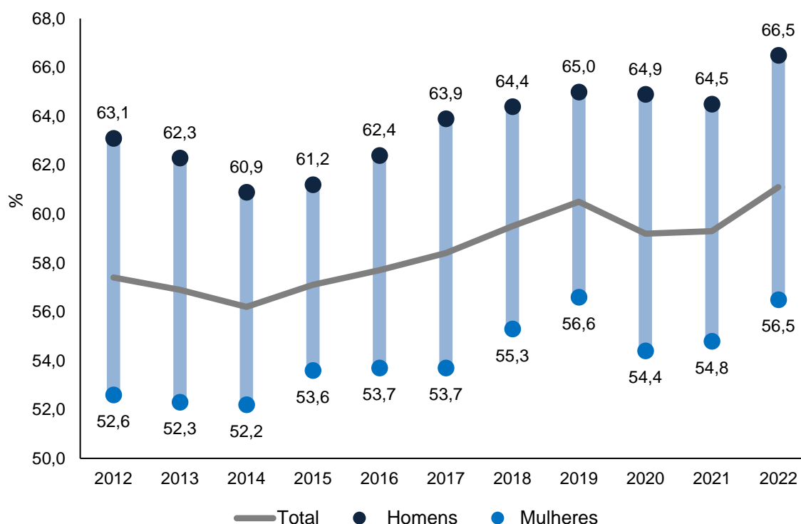
Fig. II.2 – Taxa de atividade, por sexo, 2012-2022
